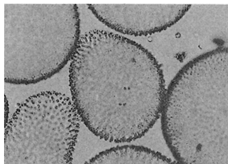
【淡水赤潮(ウログレナ・アメリカナ)】
